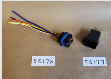
58176 - Mini Relay Connector 58177 - Mini Relay
